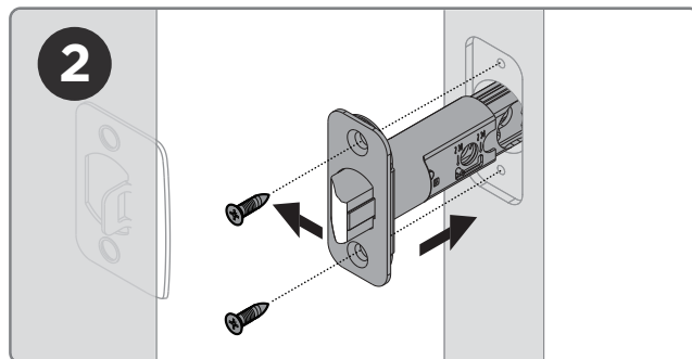
Install the latch with the slanted surface facing the strike Instale el pestillo con la superficie inclinada orientada hacia la placa Installez le loquet avec la surface inclinée tournée vers la gâche
