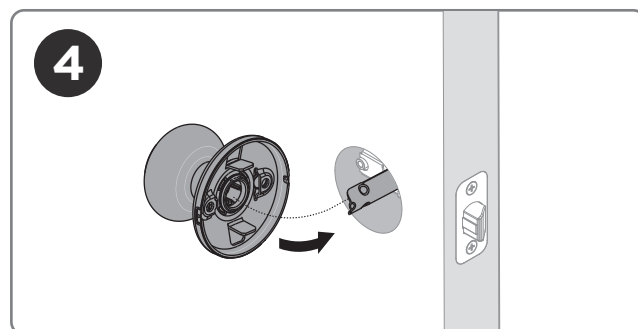
Install the interior Instale el interior Installez l'intérieur
